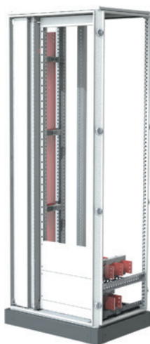
Распределительные панели с вертикальной шиной
