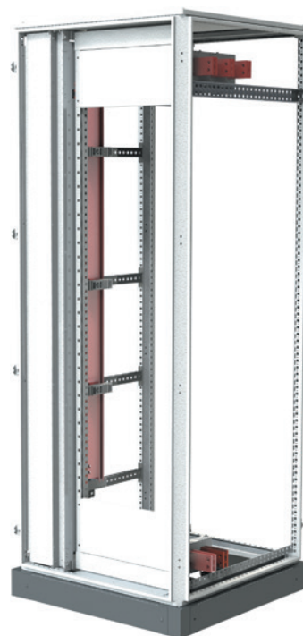
LMFD 200.80.80-2000A-OD-3-4
