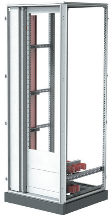
LMFD 200.80.80-2000A-OU-3-4
