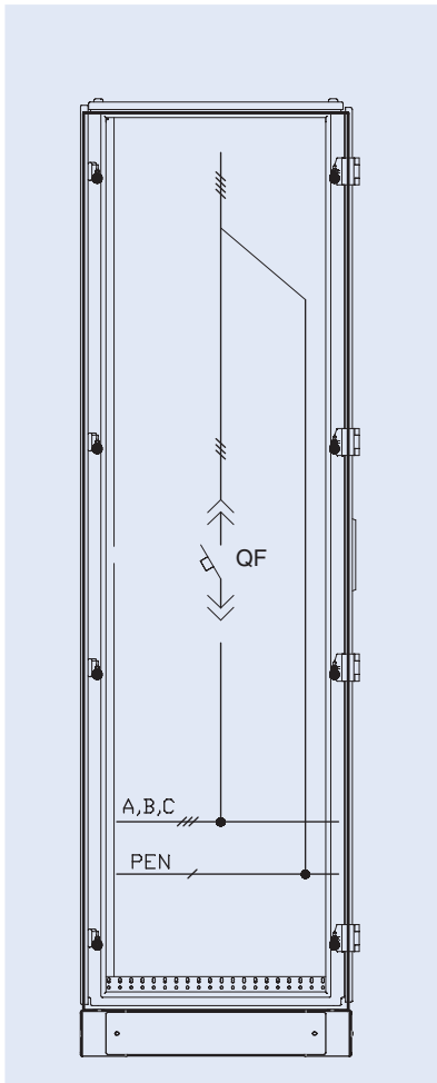
Однолинейная схема
