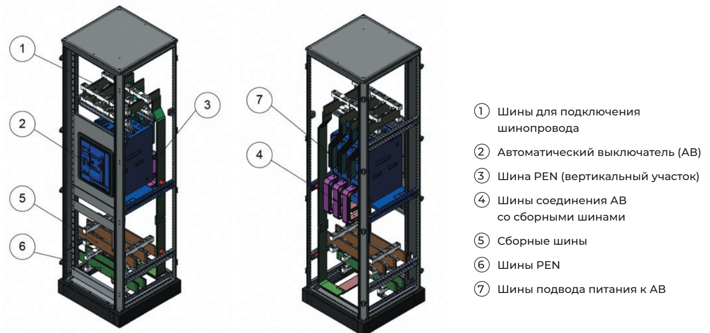
Расположение узлов схемы в конструкции шкафа ввода
