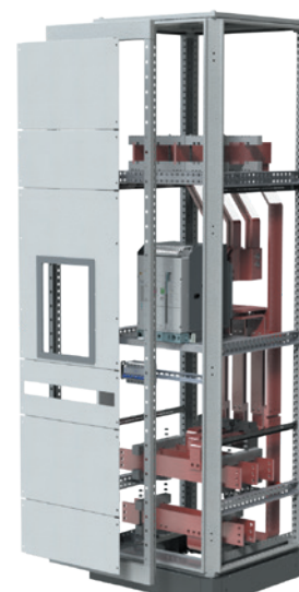
Пластронная система, автомат и шины
