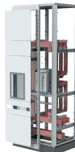
Пластронная система, автомат и шины
